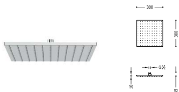
Rociador ducha anticalcárea CUB-300 Latón 300x300 mm.
