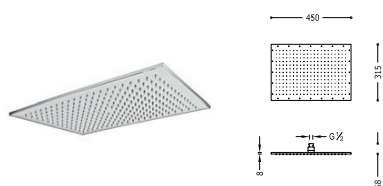
Rociador ducha anticalcárea 450x315 mm.
