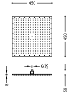
Rociador ducha anticalcárea 450x450 mm.
