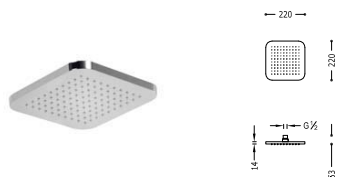
Rociador ducha anticalcárea LOFT-220 todo cromo 220x220 mm.
